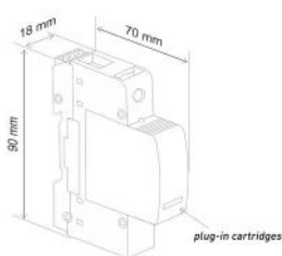
1 Pole
