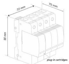
4 Poles
